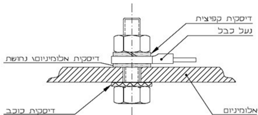
איור מספר 11 תקנות 21(ב) ו-26(ג) דוגמה לחיבור נחושת / אלומיניום
