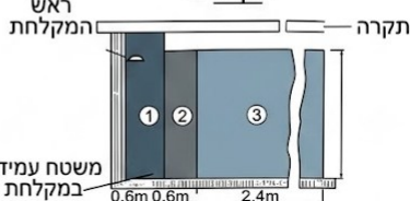
חתך א-א
